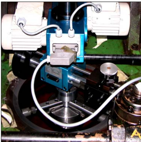
Plandrehen am Motorblock
