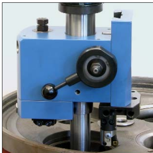
Grundbohrung ausdrehen
