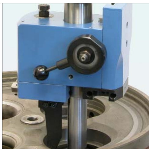
Grundbohrung plandrehen
